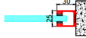
DUVAR BAŞLANGICI
